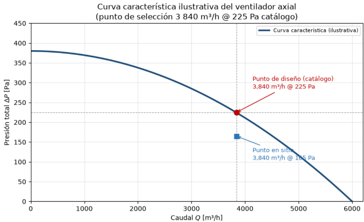
Figura 1. Curva característica ilustrativa.
